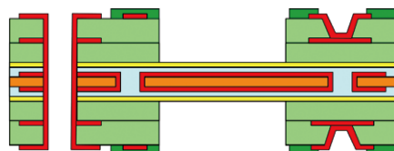
断面構造例
